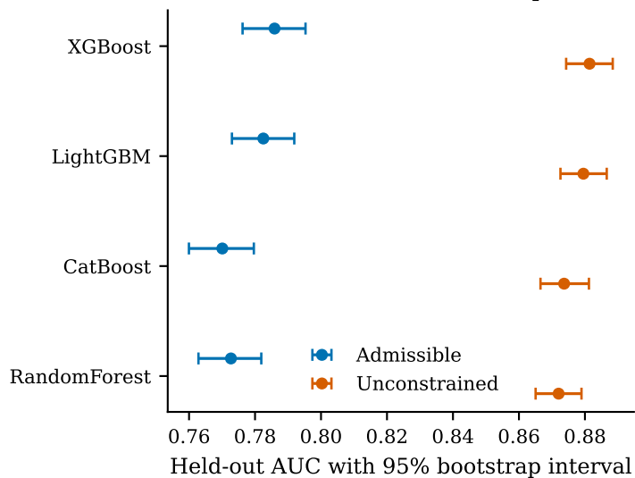
(b) Test AUC, 2000 resamples
