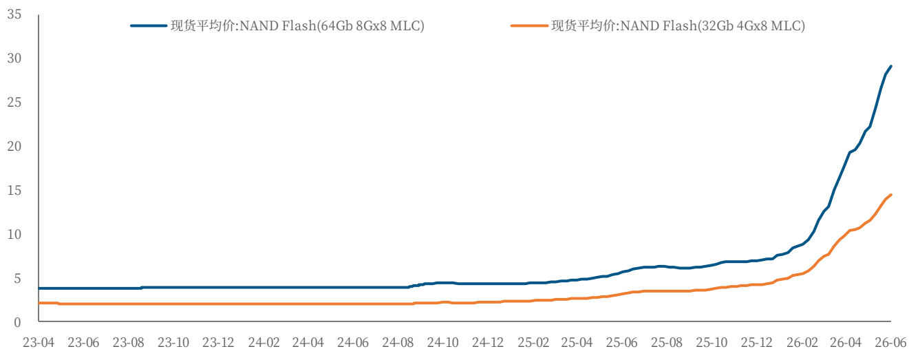
图11: NAND (32Gb/64Gb 部分产品) 价格走势/美元
