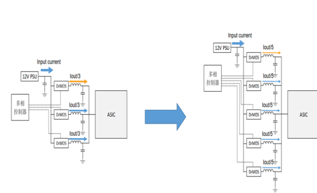
图21：DrMOS 相数扩展示意图
