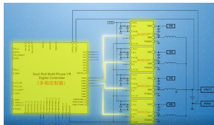
图：多相电源示例图
