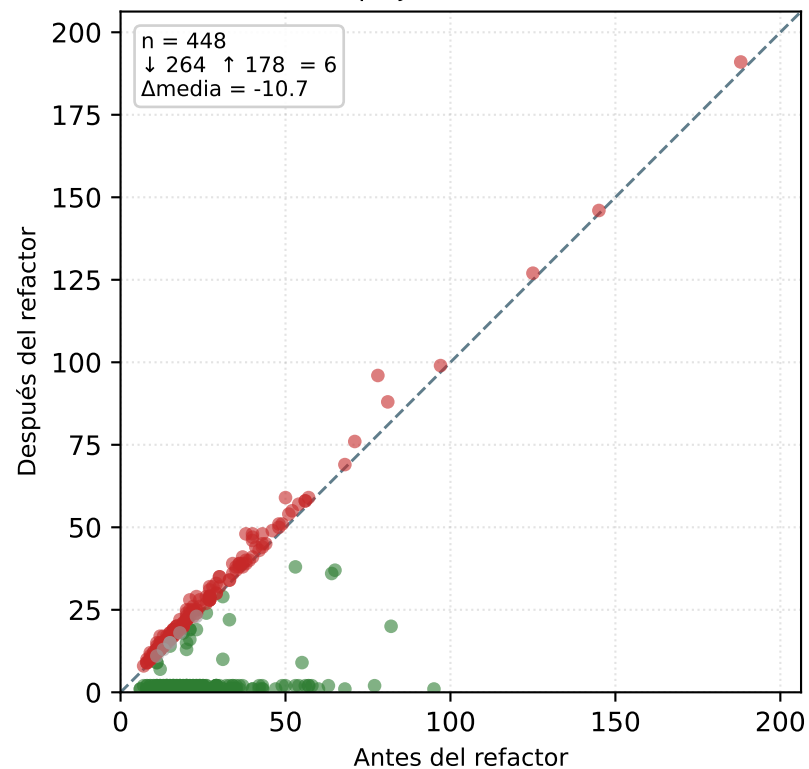
Complejidad ciclomática
