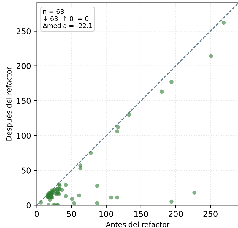
Complejidad cognitiva
