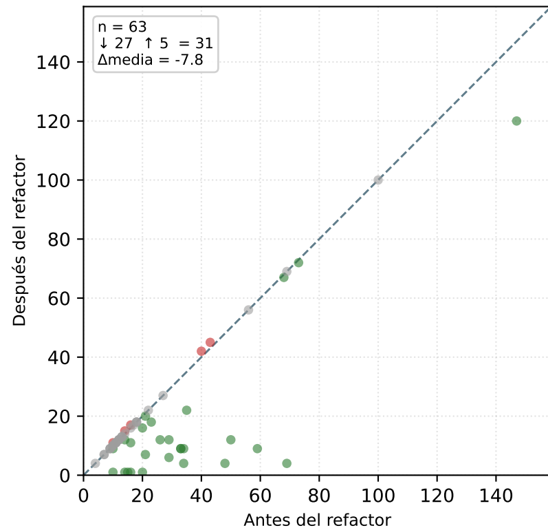
Complejidad ciclomática
