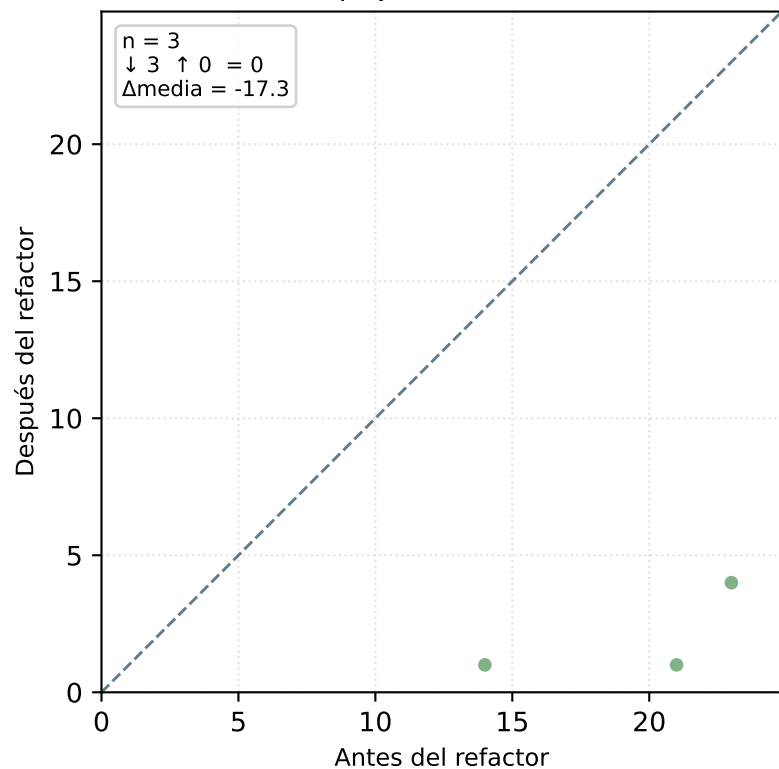
Complejidad ciclomática
