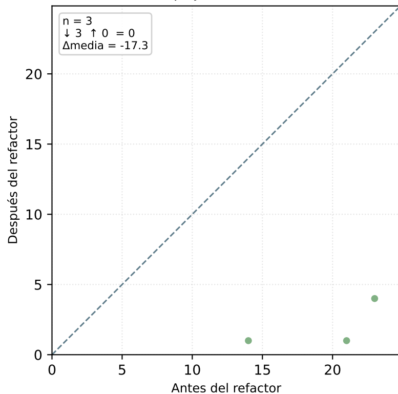
Complejidad ciclomática
