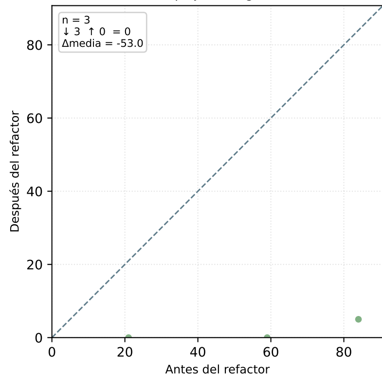
Complejidad cognitiva
