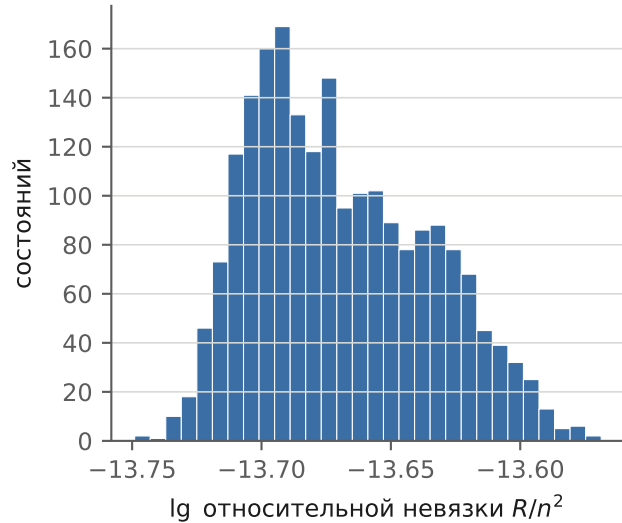
невязка факторизации, медиана 2.1\text{e-}14
