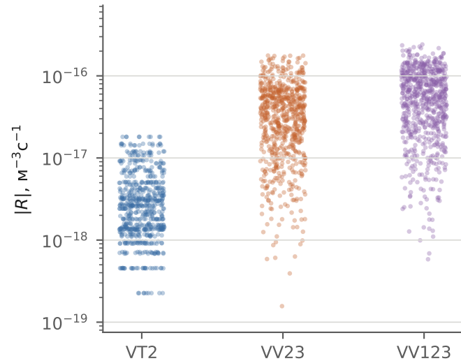
распределение |R|
