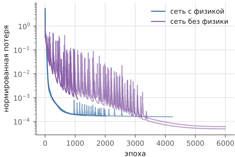
три запуска на каждую архитектуру
