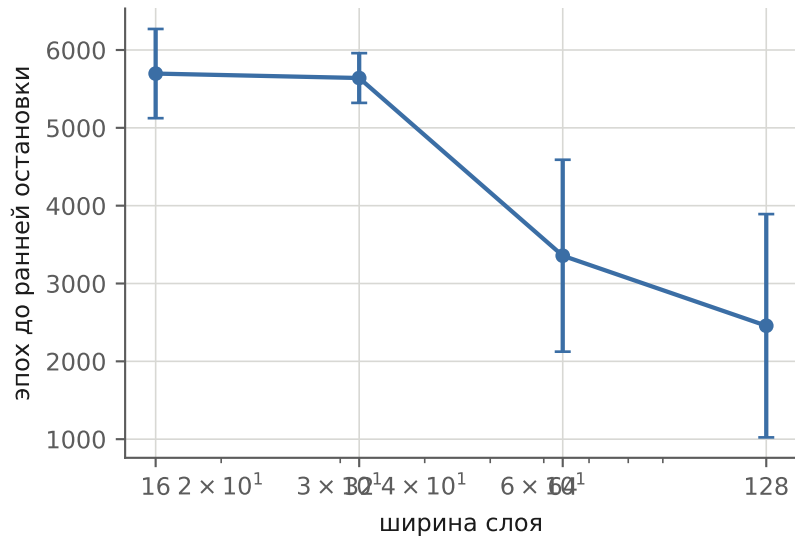
сходимость против ёмкости
