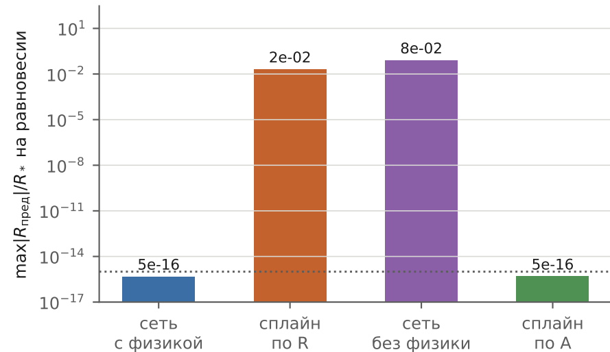
невязка равновесия R(T, T, T) = 0
