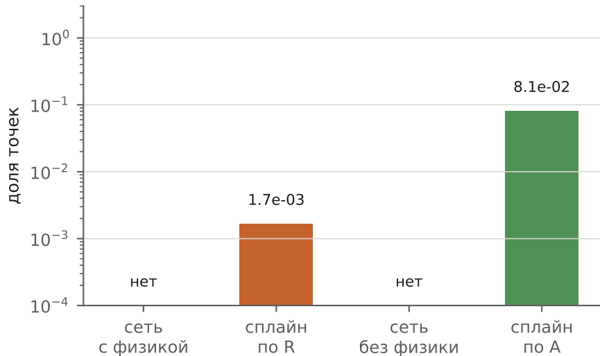
доля неверного знака R
