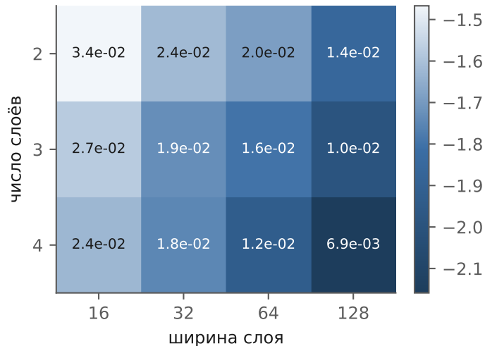
lg средней ошибки
