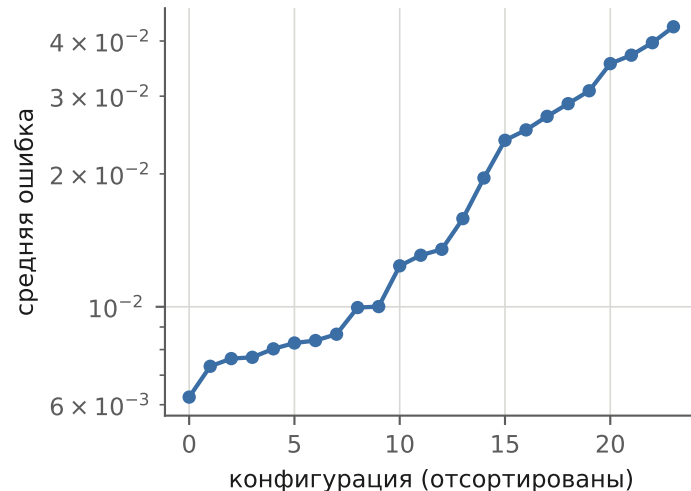
разброс по точности 6.9x
