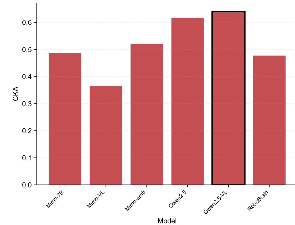
CKA
