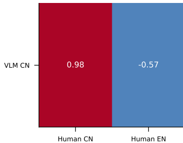
VLM
