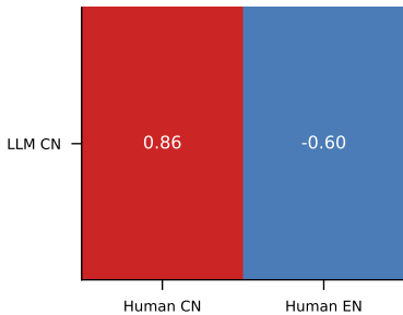
LLM
