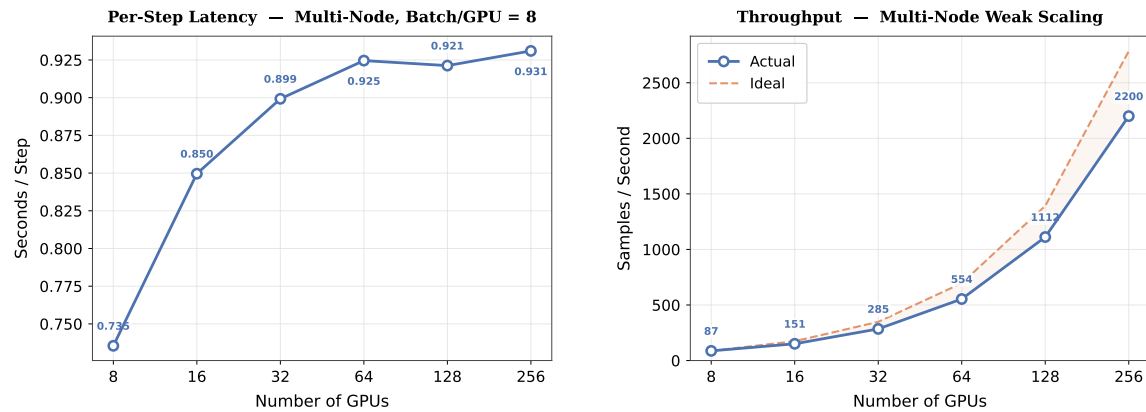
图 6: 多节点扩展效率。左图: 从 8 到 32 个 GPU, 每步延迟因节点间通信开销而显著上升, 然后在 64 到 256 个 GPU 之间趋于平稳。右图: 实测样本吞吐量与理想线性扩展的对比; 超过 32 个 GPU 后, 并行效率稳定在约 79 – 80%。
