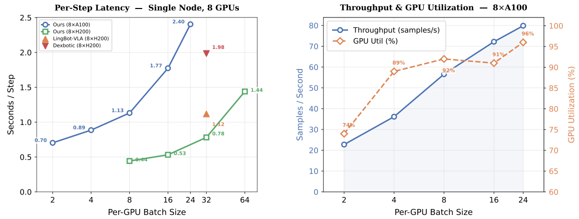
图 5: 单 8-GPU 节点上的每步延迟和吞吐量。左图: 在 A100 和 H200 上, 我们的方法每 GPU 批大小与步延迟的关系, 并与 LingBot-VLA 和 Dexbotic (均在 8 \times H200 上) 进行比较。右图: 在 8 \times A100 上不同批大小下的训练吞吐量和 GPU 利用率。
