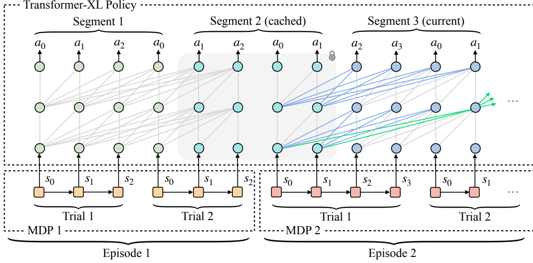
图 3: 为了实现长上下文适应, 我们允许局部变换器 (LocoFormer) 关注先前试验中的状态。我们采用长上下文变换器 (Transformer) 骨干网络, 将上下文划分为固定长度的片段。在处理当前片段时, 键和值也从前一个 (缓存的) 片段中的状态计算得出, 但梯度不会传播 (蓝色线条)。随着层数的增加, 这使得局部变换器甚至能够利用缓存片段之前的片段中的信息 (绿色线条)。
