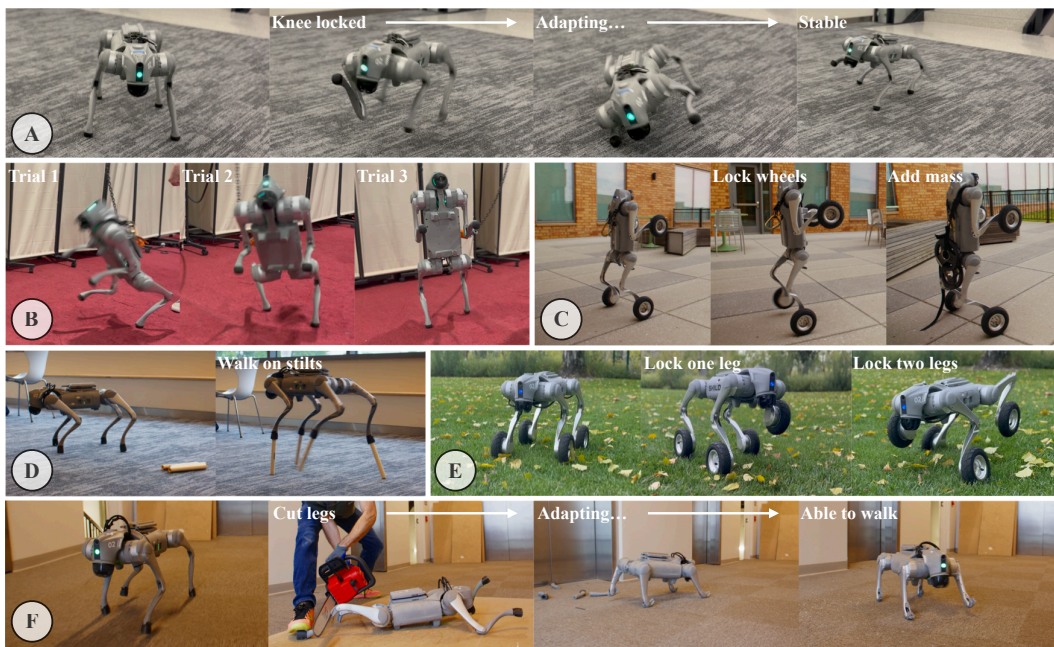
图 5：我们展示了涌现的适应行为，全部来自同一个 LocoFormer 模型。A：一个膝盖被锁定，LocoFormer 适应用剩余三条腿行走。这不是训练的一部分。B：如果 LocoFormer 在一次试验中无法适应，它会保留之前试验的记忆并提高性能。C：轮子被锁定，LocoFormer 检测到突然变化，并切换到行走步态。当附加质量时，LocoFormer 也能适应。D：安装了高跷，LocoFormer 适应延长的腿长以继续行走。E：在一条或两条腿被锁定的情况下，LocoFormer 调整其运动以保持平衡。F：小腿被截断后，机器人在数十秒后适应用膝盖行走，尽管在训练时从未见过这种情况。
