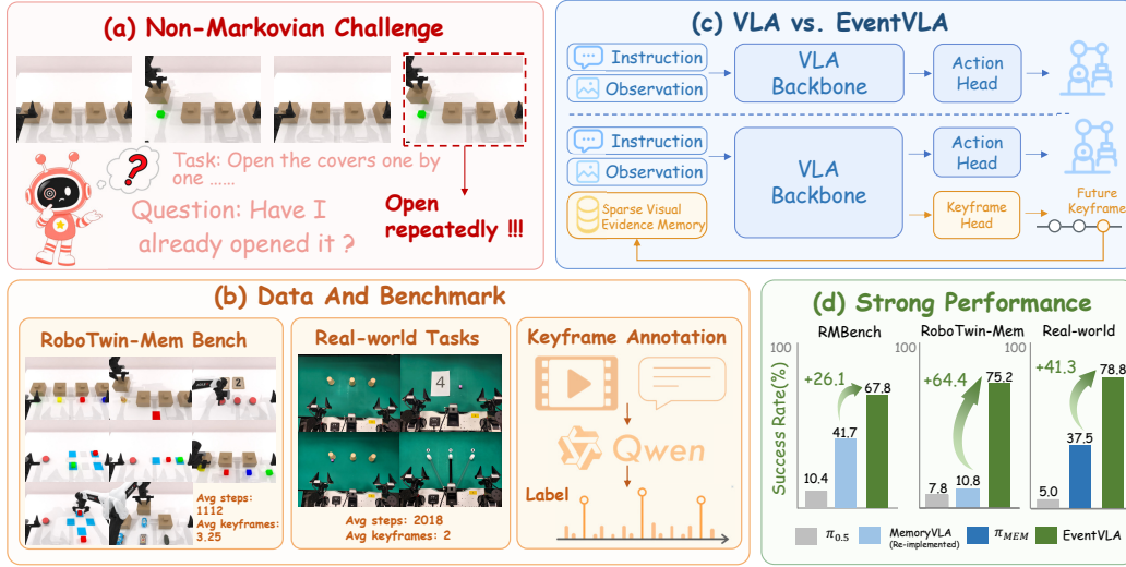
图 1: EventVLA 概览。EventVLA 通过存储稀疏、任务关键的视觉证据来处理长时程、需要记忆的操作任务。该图展示了 (a) 非马尔可夫挑战, (b) 我们提出并评估的基准, (c) 事件驱动的记忆设计, 以及 (d) 在仿真与真实世界任务中的显著提升。
