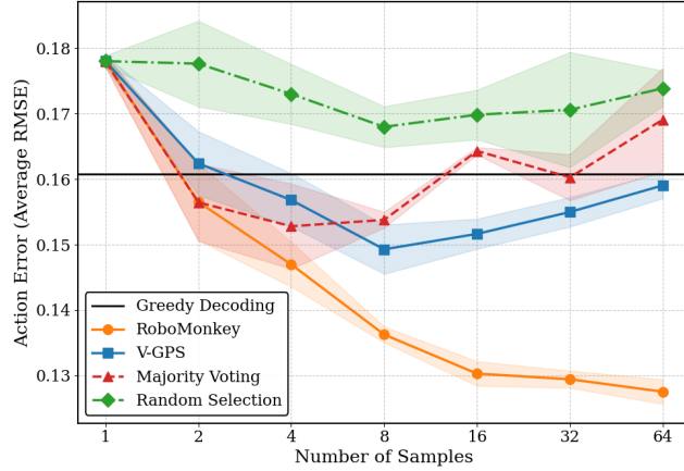
图 8: 不同选择方法在生成样本数量增加时的动作误差（平均均方根误差）比较。RoboMonkey 持续优于其他基线，并能有效利用额外计算资源进行扩展。
