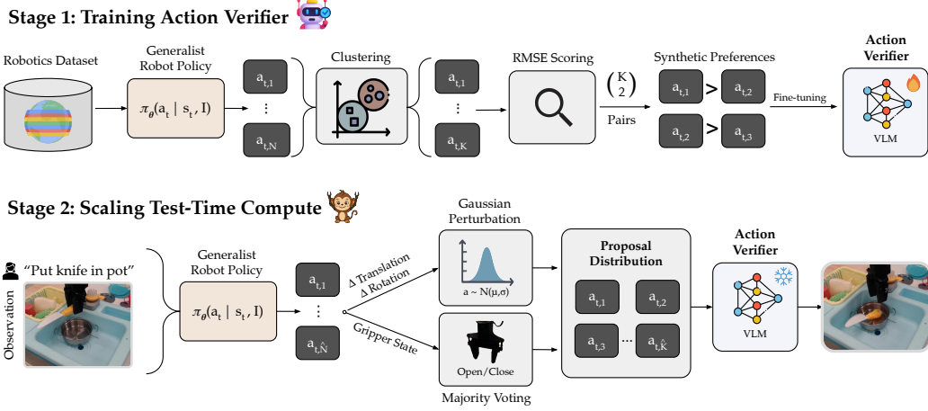
图 2：阶段 1：训练动作验证器。 给定模仿学习数据集，我们从通用机器人策略中为每个状态采样 N 个候选动作，并应用聚类将其缩减为 K 个代表性动作。我们构建 \binom{K}{2} 个合成动作比较，并根据每个采样动作与真实动作之间的均方根误差分配偏好。该合成偏好数据集随后用于微调基于视觉语言模型的动作验证器。阶段 2：扩展测试时计算。在部署时，我们根据给定的任务指令和观测从通用机器人策略中采样 N 个初始动作。我们对这些动作的平移和旋转分量 ( \Delta x, \Delta y, \Delta z, \Delta u, \Delta v, \Delta w )，如第 2 节所述) 拟合高斯分布 \mathcal{N}(\mu, \sigma) ，并使用多数投票确定夹爪状态。这创建了一个动作提议分布，我们可以从中高效采样候选动作，开销可忽略不计。最后，我们使用微调后的基于视觉语言模型的验证器评估这些 K 个候选动作，并选择最优动作。
