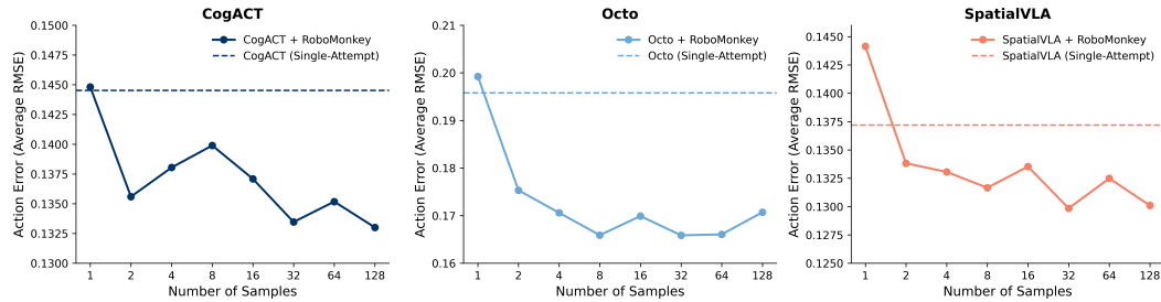
图 9: RoboMonkey 在不同通用机器人策略下扩展测试时计算的效果。动作误差（平均均方根误差）随样本数量增加而降低。虚线表示各基础策略仅生成单个动作时的动作误差。
