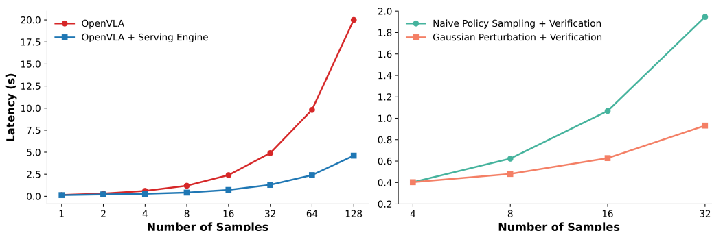
图 5: 左: 重复采样可以利用键值缓存优化和批处理, 实现比贪心解码更高的吞吐量。因此, 我们扩展了 SGLang 的能力, 以正确支持 OpenVLA。我们的优化实现显著优于朴素的 OpenVLA 推理流程, 在不同批大小下实现了更低的延迟和显著更高的吞吐量。右: 随着采样数量的增加, 朴素策略采样与高斯扰动之间的延迟比较。
