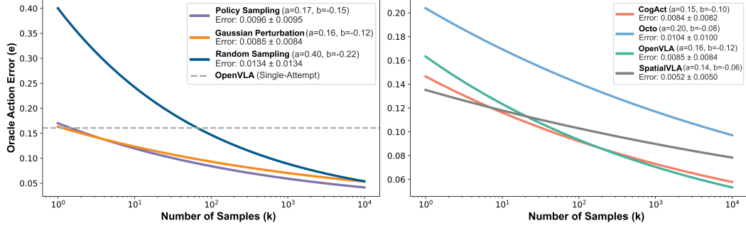
图 1：推理时缩放定律： 我们观察到，在存在理想验证器的假设下，随着生成动作数量的增加，动作误差在多种采样方法下均持续下降。从机器人策略中重复采样动作、对少量采样动作施加高斯扰动，甚至随机采样，均优于单次尝试的 OpenVLA。我们还发现，通过高斯扰动生成的样本数量与动作误差之间的关系在多种 VLA 模型（包括 CogACT、Octo、OpenVLA 和 SpatialVLA）上近似遵循幂律。对于幂律拟合，我们将动作误差的对数 e 建模为样本数量 k : \log(e) \approx \log(a) + b \cdot \log(k) 的函数，其中 a 和 b 为拟合的模型参数。
