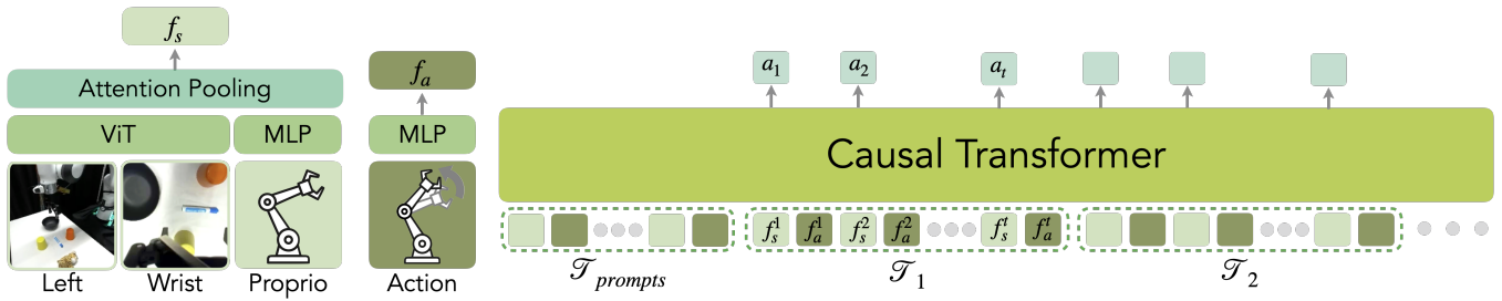
图 3：方法概览： （左）我们使用预训练的视觉变换器对相机观测进行编码。此外，我们使用多层感知机对本体感觉进行编码。我们将视觉潜变量与本体感觉潜变量拼接，并使用注意力池化提取特征 f_s 作为当前状态表示。我们使用多层感知机对当前动作进行编码，得到 f_a 。（右）我们将同一任务的多个轨迹拼接，并随机采样前 k 条轨迹作为提示。因果变换器自回归地预测下一系列令牌。我们解码位于状态特征位置的令牌，通过多层感知机生成下一个 h = 16 动作。
