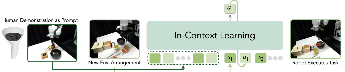
图 1：上下文机器人变换器 (ICRT)：一种具备上下文模仿学习能力的机器人基础模型。ICRT 在大规模感觉运动轨迹上进行下一词元预测。在推理时，它以人类遥操作演示的原始感觉运动轨迹作为提示，使模型能够执行新任务并实现实时连续控制，无需微调。
