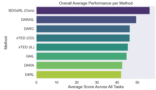
图 2: 各方法在所有任务、领域差距和演示级别上的总体平均性能。
