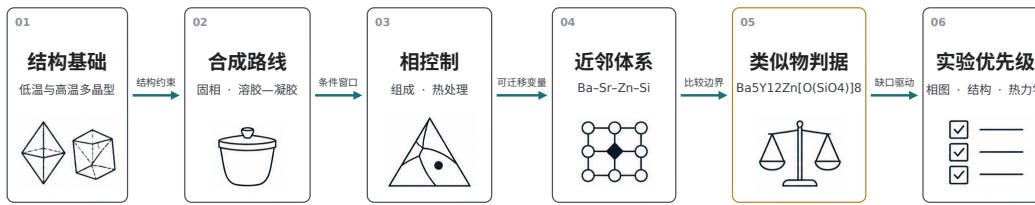
图 1: 本文的行文路线图。箭头表示从结构事实到合成窗口、结构相关化合物规律的迁移和可证伪实验建议的推进顺序。
