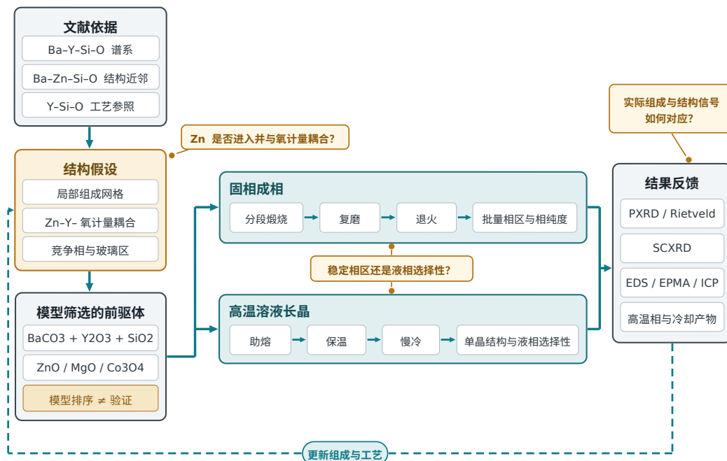
图 1: 本文的研究路线。 Ba-Y-Si-O、Ba-Zn-Si-O 和 Y-Si-O 体系先用于确定结构关系、竞争相和工艺边界；相图与电荷平衡分析提出候选组成，两步无机逆合成模型给出前驱体集合；固相反应与高温溶液法晶体生长分别考察块体相区和单晶结构，表征结果用于调整后续的组成和工艺。
