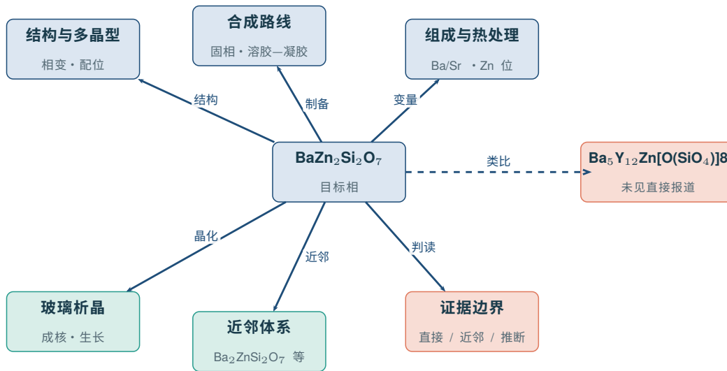
图 2: \text{BaZn}_2\text{Si}_2\text{O}_7 合成与相控制的分类框架。实线分支表示目标相的直接实验依据或结构相关化合物的实验依据，虚线节点表示尚无直接结构报道的比较对象。
