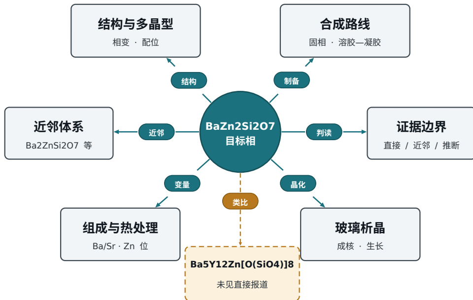
图 2: \text{BaZn}_2\text{Si}_2\text{O}_7 合成与相控制的分类框架。实线分支表示目标相的直接实验依据或结构相关化合物的实验依据，虚线节点表示尚无直接结构报道的比较对象。
