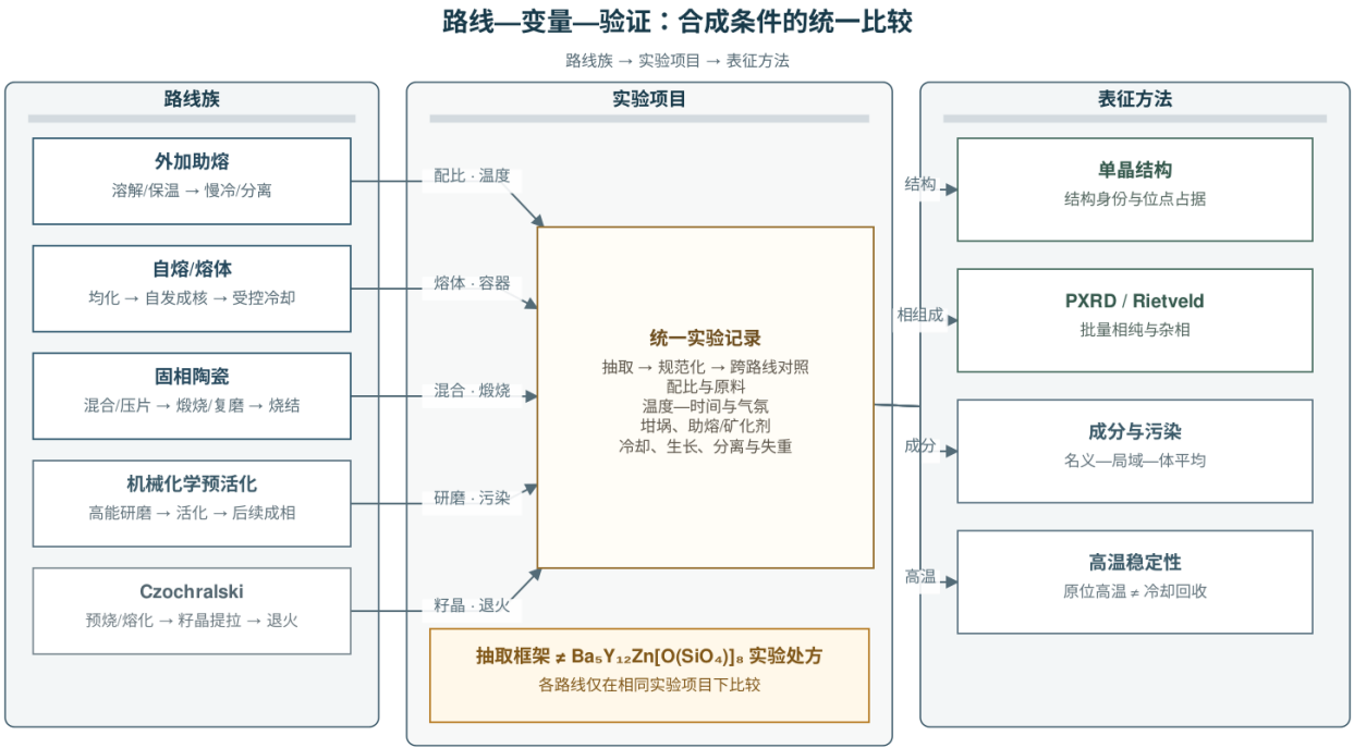
图 3 不同合成方法的条件比较与产物表征。左侧区分外加助熔、自熔/熔体、固相陶瓷、机械化学预活化和 Czochralski 路线；中部列出可比较的原料、热历史、气氛、容器、冷却和生长条件；右侧列出单晶结构、PXRD/Rietveld 精修、成分分析及高温稳定性等互补表征。连线表示实验条件与表征结果的对应关系，不表示变量与相形成之间的因果关系；Czochralski 路线仅作工艺参照，本图不构成目标相的实验配方。
