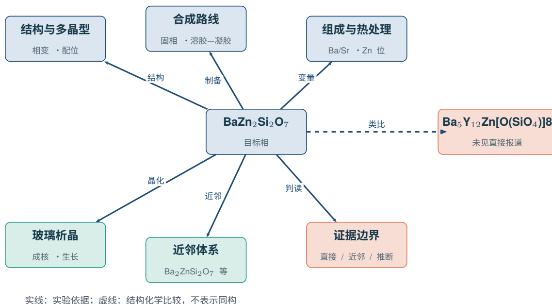
图 2. \text{BaZn}_2\text{Si}_2\text{O}_7 合成与相控制的分类框架。实线分支表示目标相的直接实验依据或结构相关化合物的实验依据，虚线节点表示尚无直接结构报道的比较对象。
