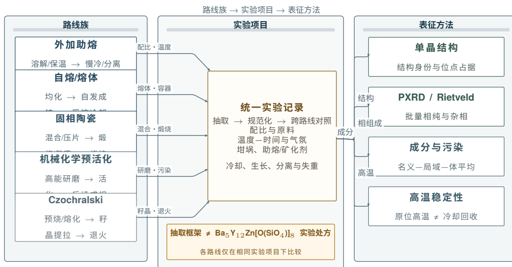
图 3. 不同合成方法的条件比较与产物表征。 左侧区分外加助熔、自熔/熔体、固相陶瓷、机械化学预活化和 Czochralski 路线；中部列出可比较的原料、热历史、气氛、容器、冷却和生长条件；右侧列出单晶结构、PXRD/Rietveld 精修、成分分析及高温稳定性等互补表征。连线表示实验条件与表征结果的对应关系，不表示变量与相形成之间的因果关系；Czochralski 路线仅作工艺参照，本图不构成目标相的实验配方。
