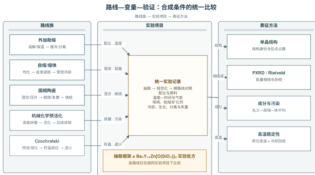
图 3: 不同合成方法的条件比较与产物表征。左侧区分外加助熔、自熔/熔体、固相陶瓷、机械化学预活化和 Czochralski 路线；中部列出可比较的原料、热历史、气氛、容器、冷却和生长条件；右侧列出单晶结构、PXRD/Rietveld 精修、成分分析及高温稳定性等互补表征。连线表示实验条件与表征结果的对应关系，不表示变量与相形成之间的因果关系；Czochralski 路线仅作工艺参照，本图不构成目标相的实验配方。
