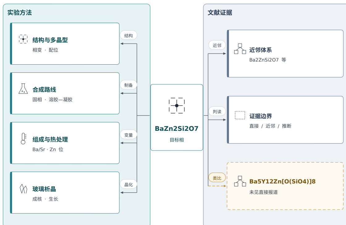
图 2. BaZn 2 Si 2 O 7 合成与相控制的分类框架。实线分支表示目标相的直接实验依据或结构相关化合物的实验依据，虚线节点表示尚无直接结构报道的比较对象。
