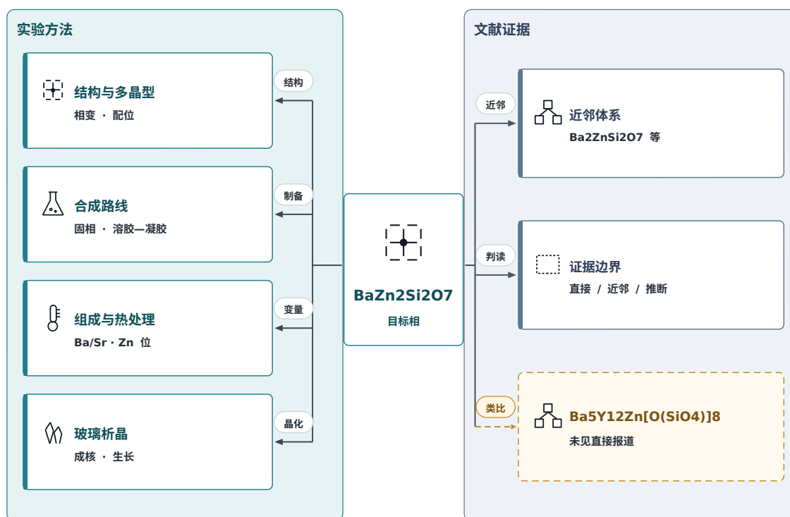
图 2. BaZn 2 Si 2 O 7 合成与相控制的分类框架。实线分支表示目标相的直接实验依据或结构相关化合物的实验依据，虚线节点表示尚无直接结构报道的比较对象。
