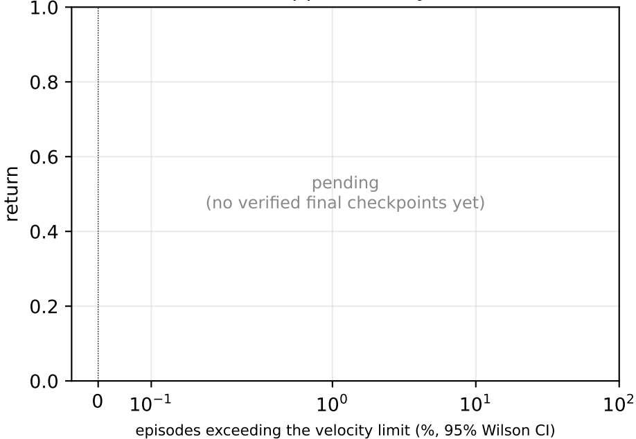
AntVelocity
