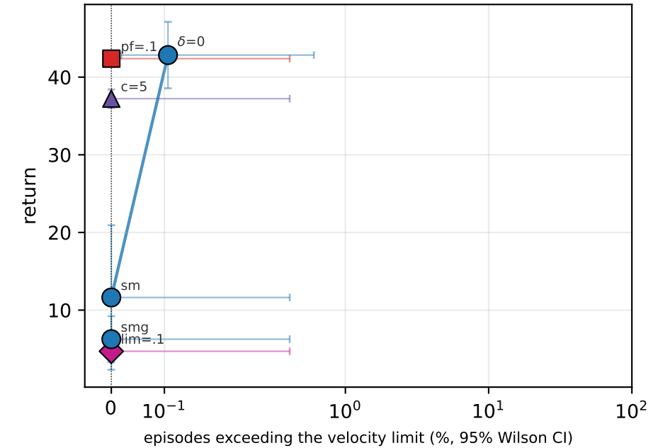
HumanoidVelocity
