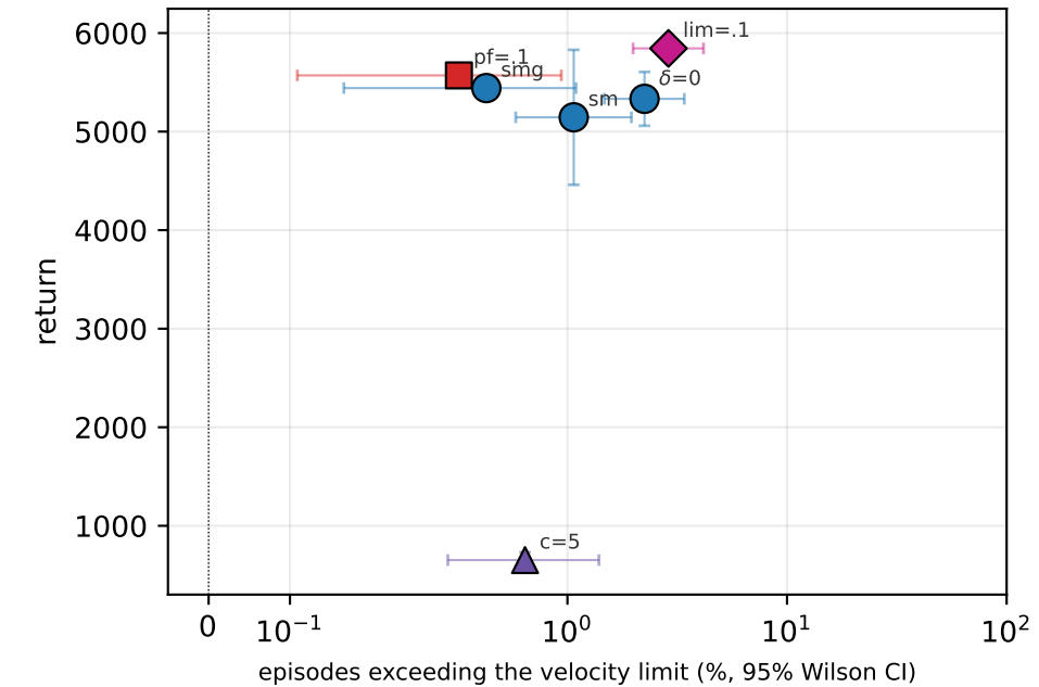
HumanoidVelocity
