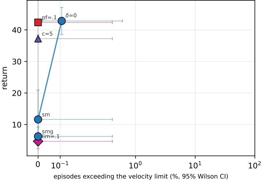
HumanoidVelocity
