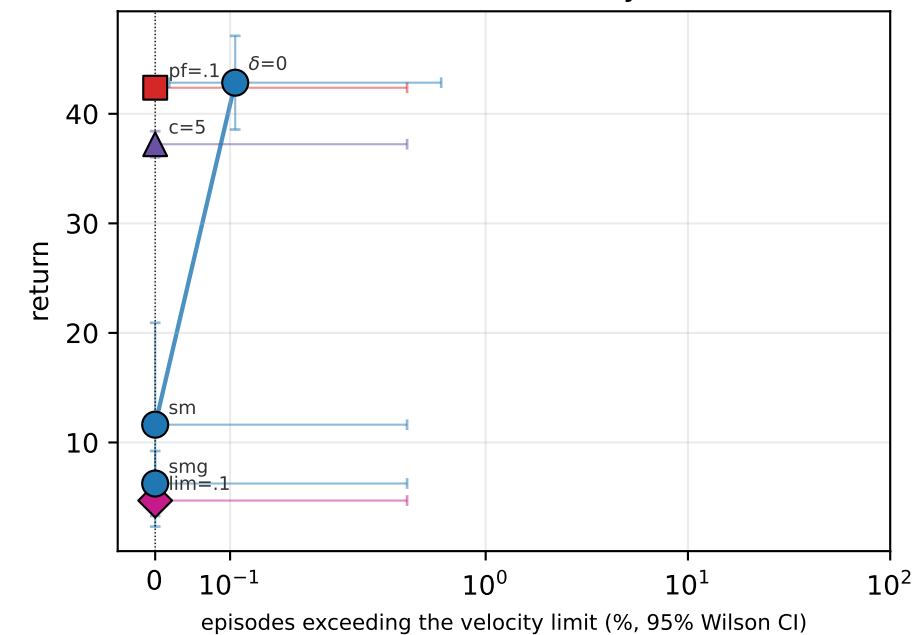
HumanoidVelocity
