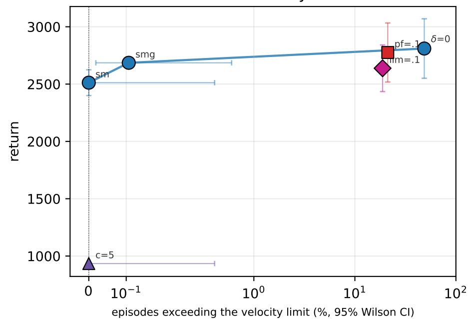
AntVelocity
