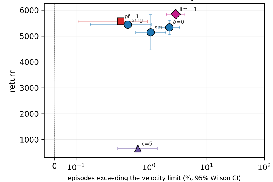
HumanoidVelocity
