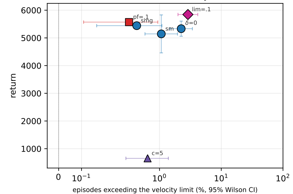
HumanoidVelocity
