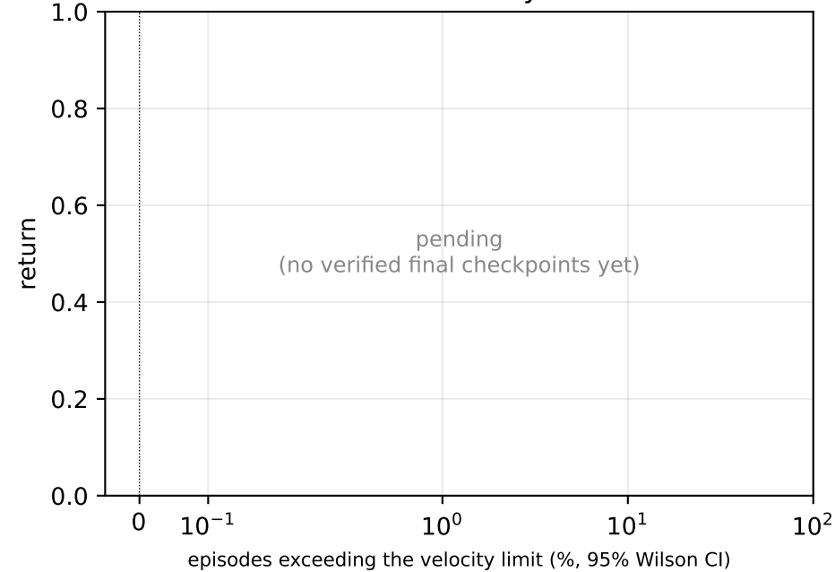
AntVelocity
