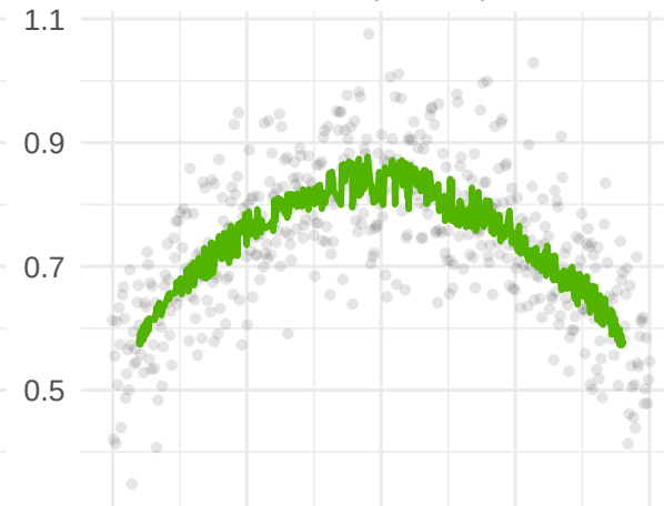
Nadaraya-Watson
