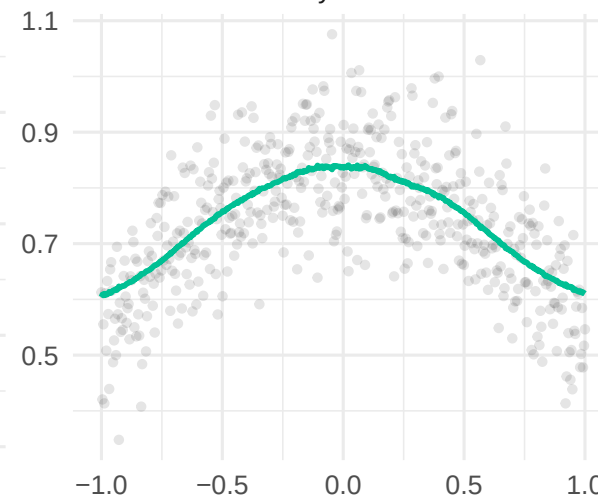
Nadaraya-Watson
