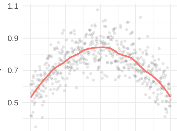
LOESS
