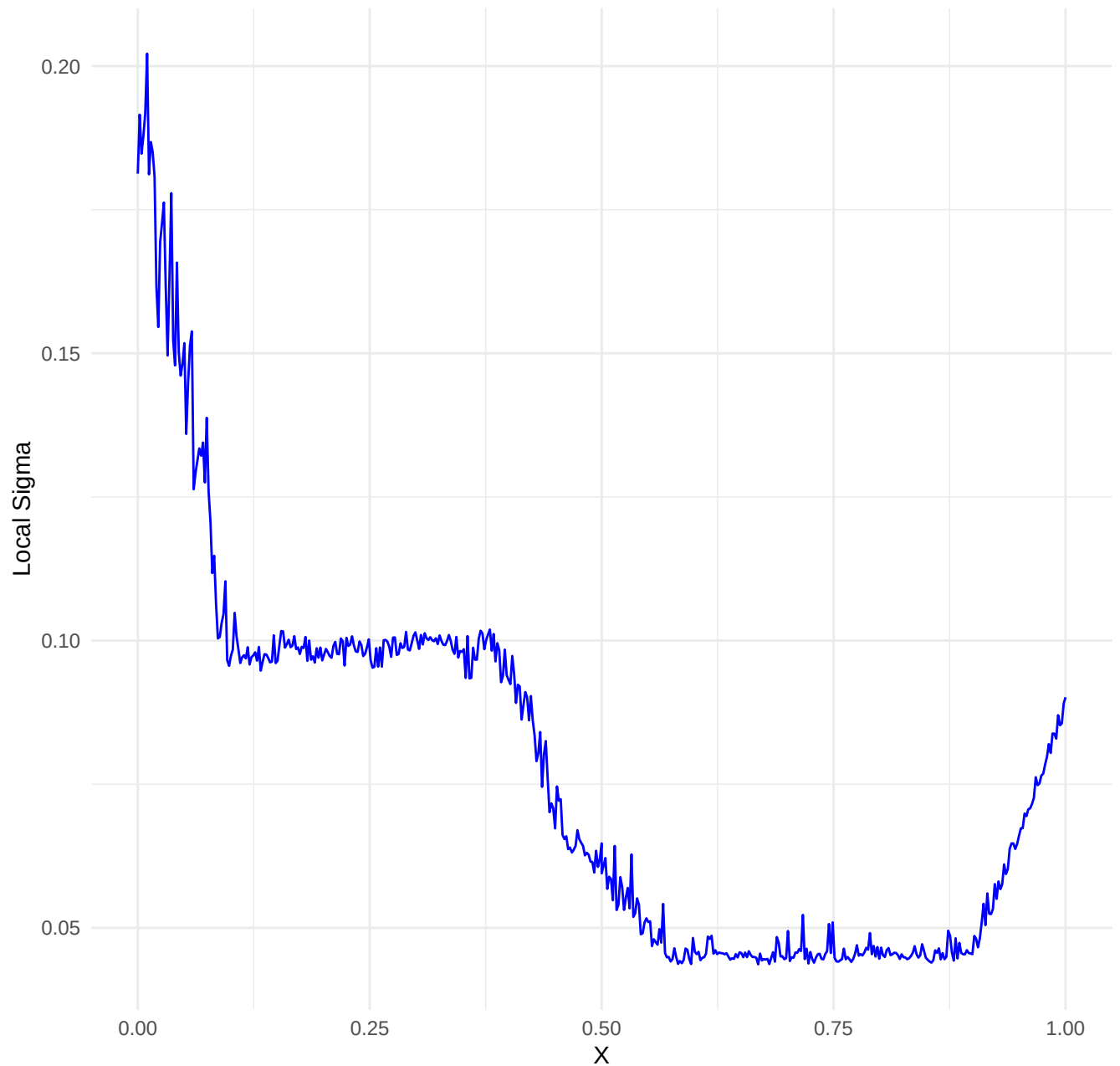
Dataset: kinked_curve_noise_low | k= 200 , iter= 21
