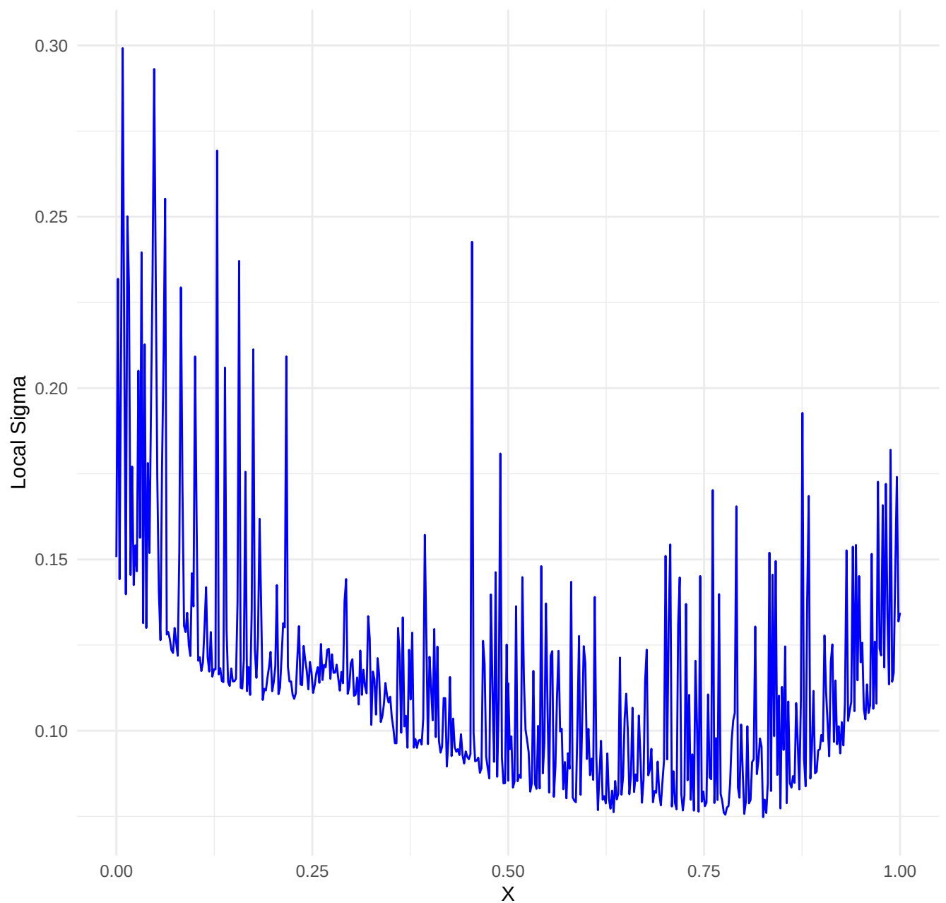
Dataset: kinked_curve_noise_high | k= 200 , iter= 21
