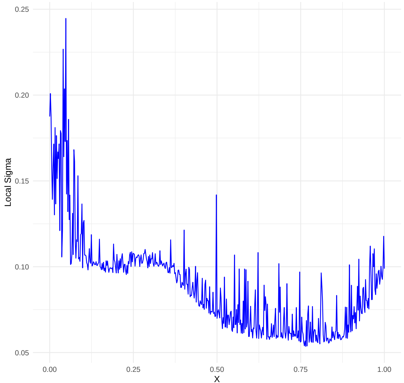
Dataset: kinked_curve_noise_medium | k= 200 , iter= 21
