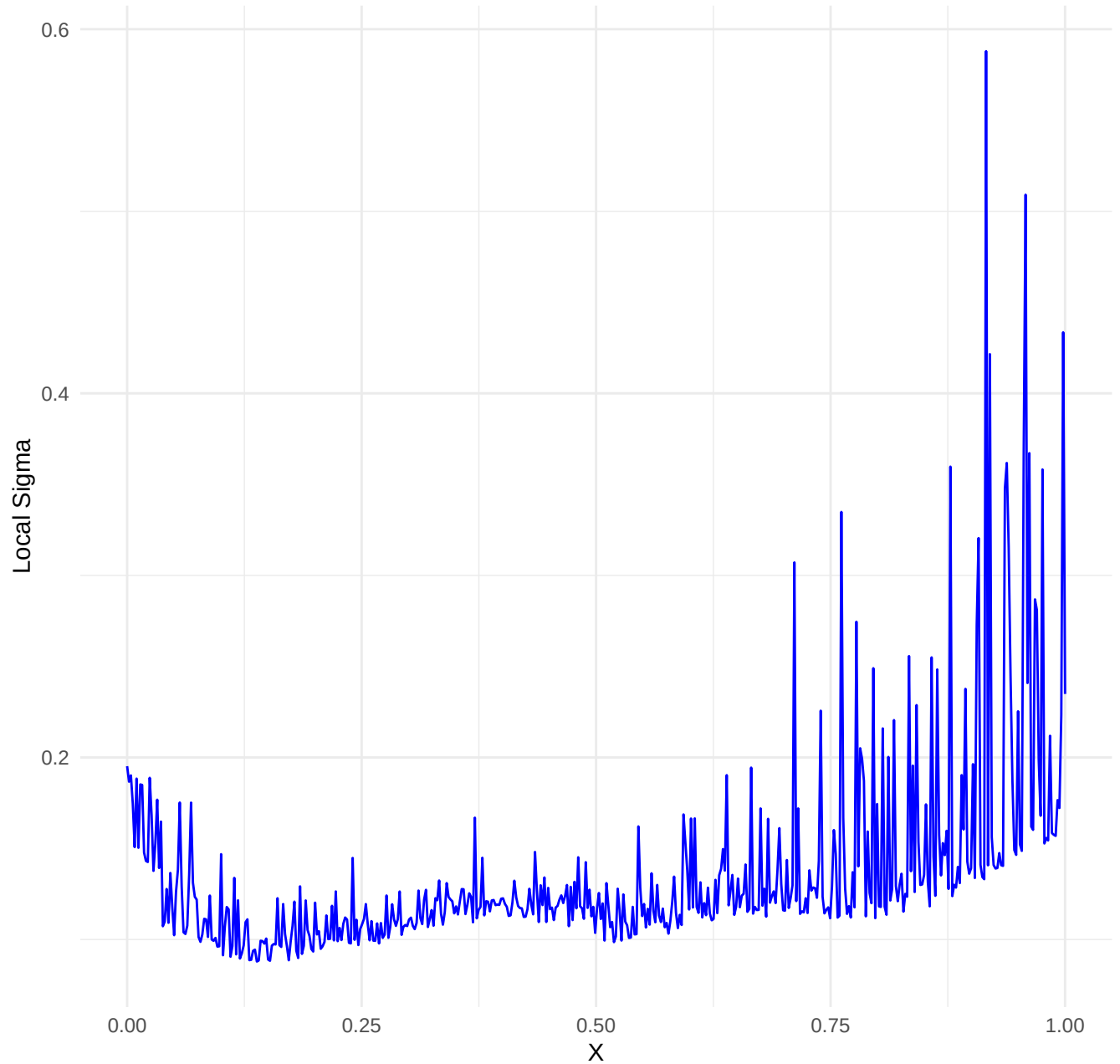
Dataset: heteroscedastic_noise_high | k= 200 , iter= 21
