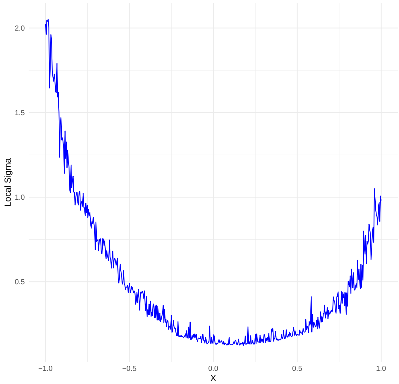
Dataset: cubic_noise_high | k= 200 , iter= 21
