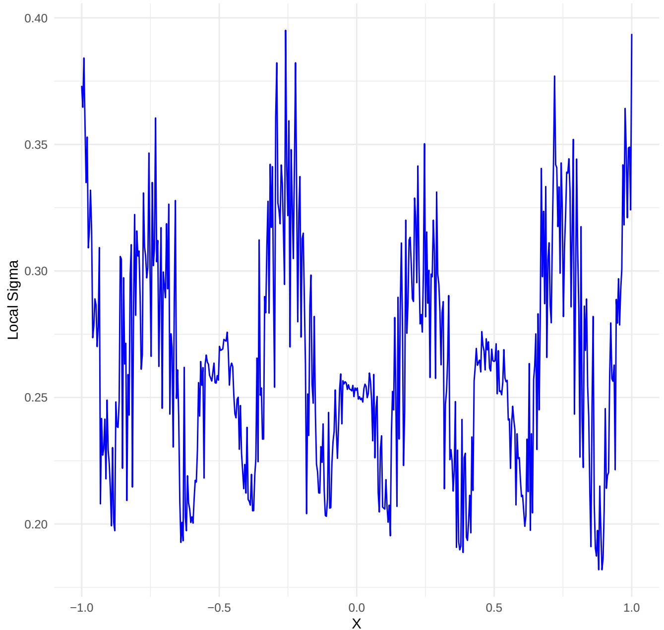
Dataset: s_curve_noise_medium | k= 200 , iter= 21
