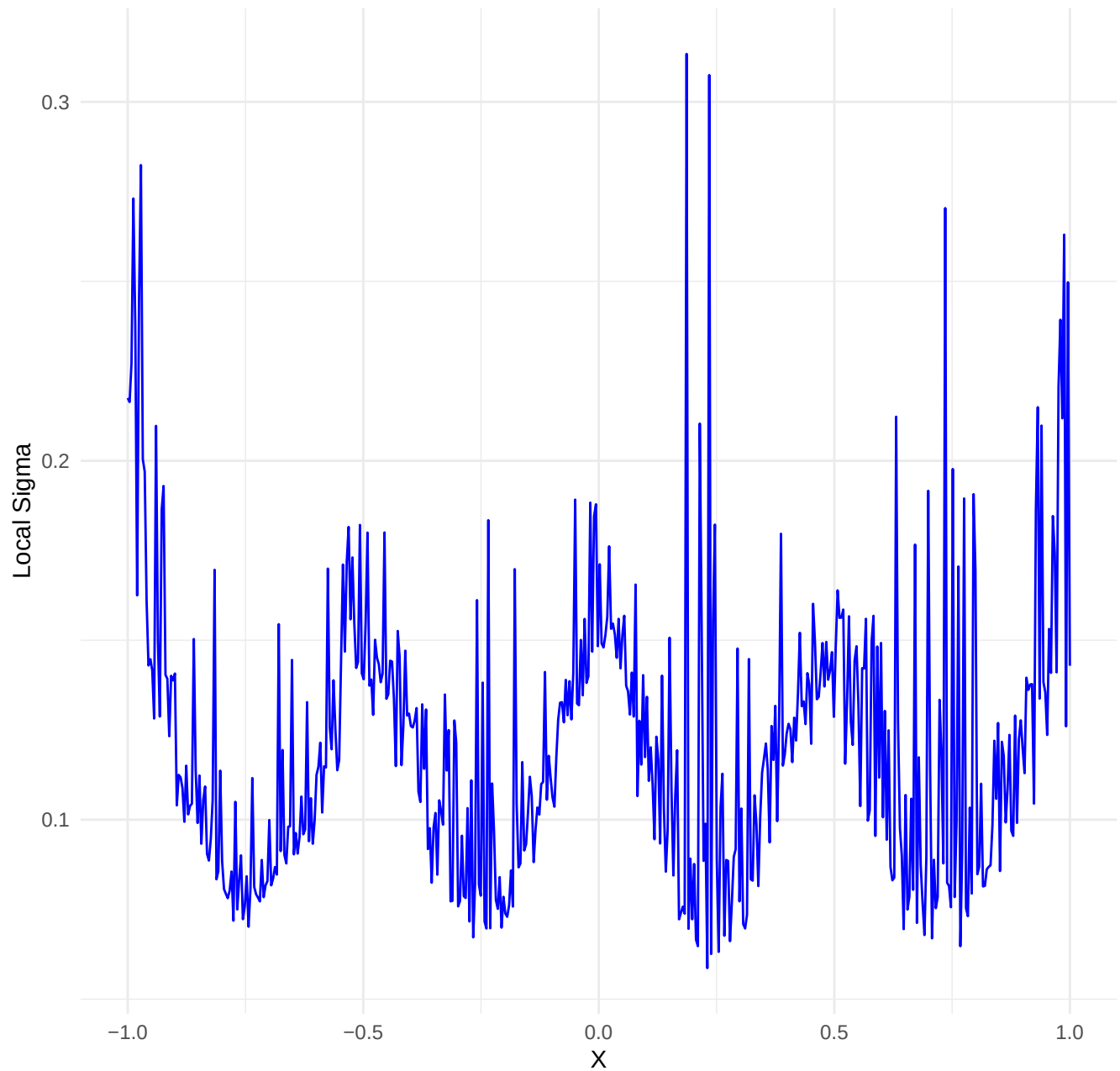
Dataset: s_curve_noise_high | k= 50 , iter= 21
