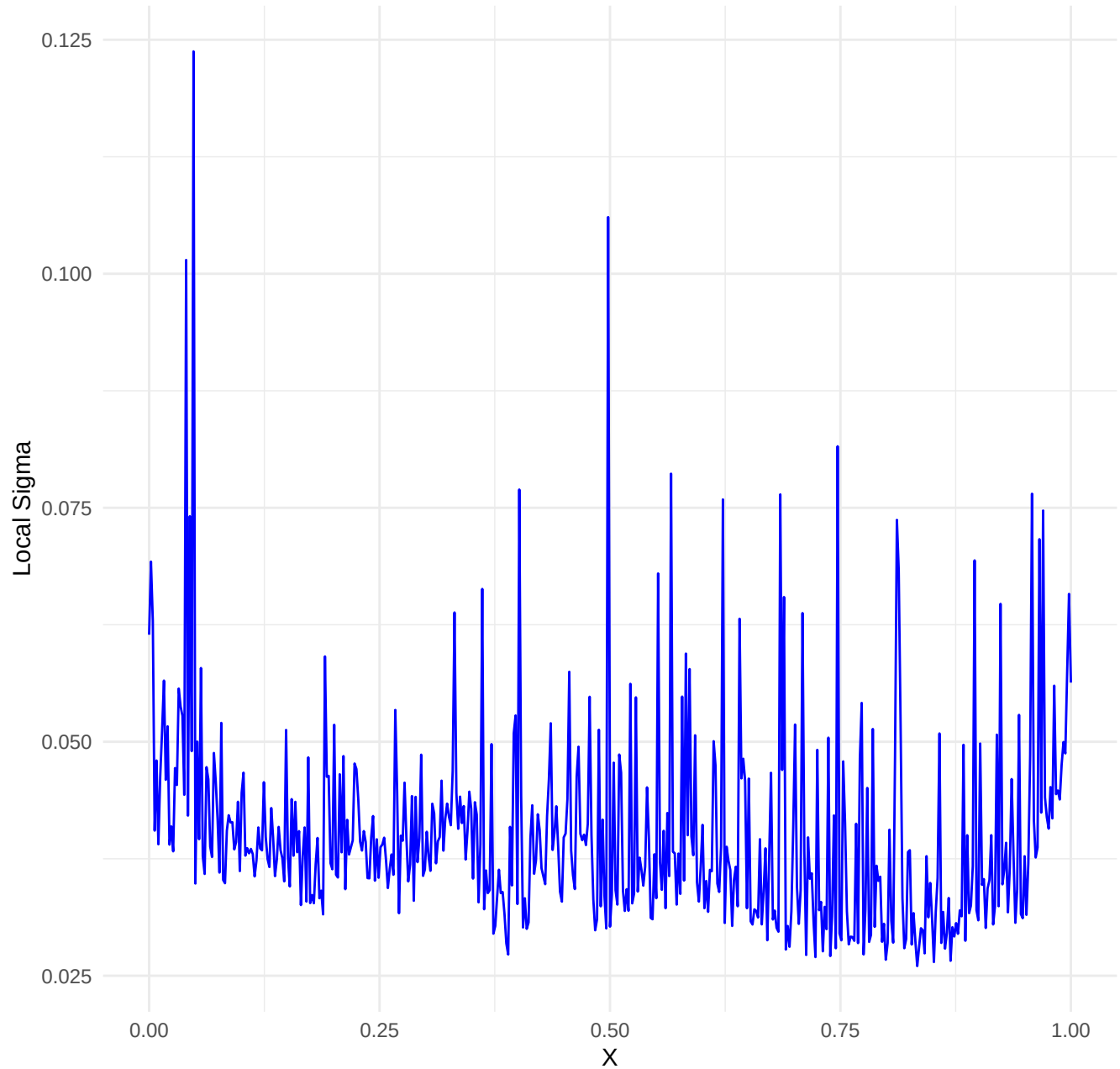
Dataset: kinked_curve_noise_medium | k= 50 , iter= 21
