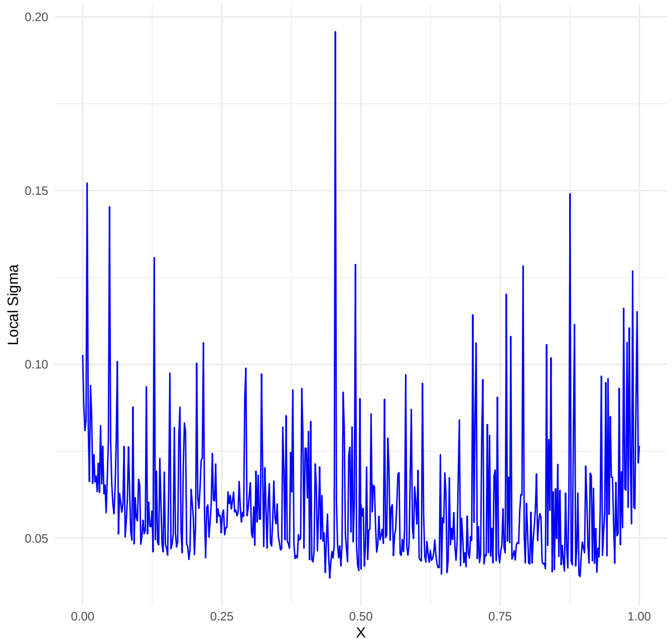
Dataset: kinked_curve_noise_high | k= 50 , iter= 21
