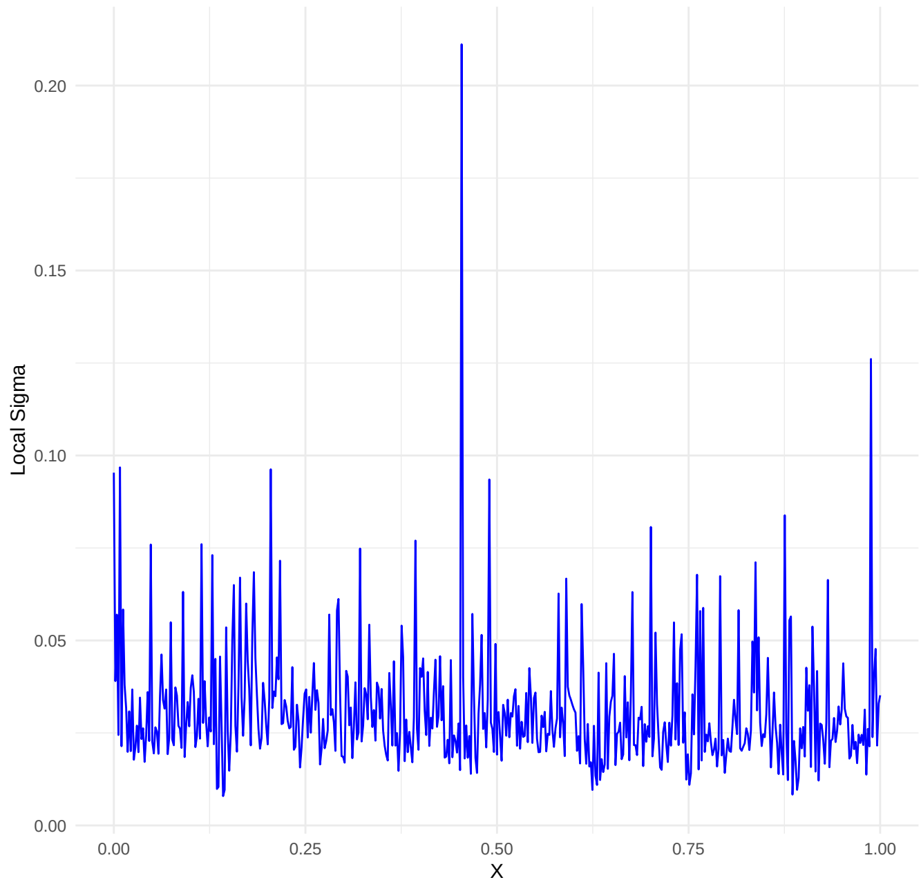
Dataset: kinked_curve_noise_high | k= 5 , iter= 21
