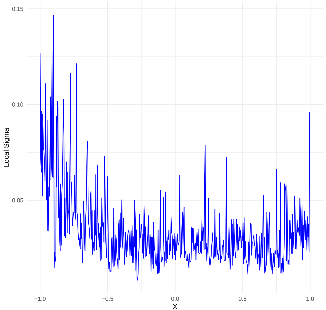
Dataset: cubic_noise_medium | k= 5 , iter= 21
