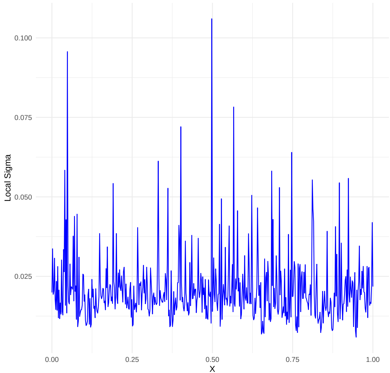
Dataset: kinked_curve_noise_medium | k= 5 , iter= 21
