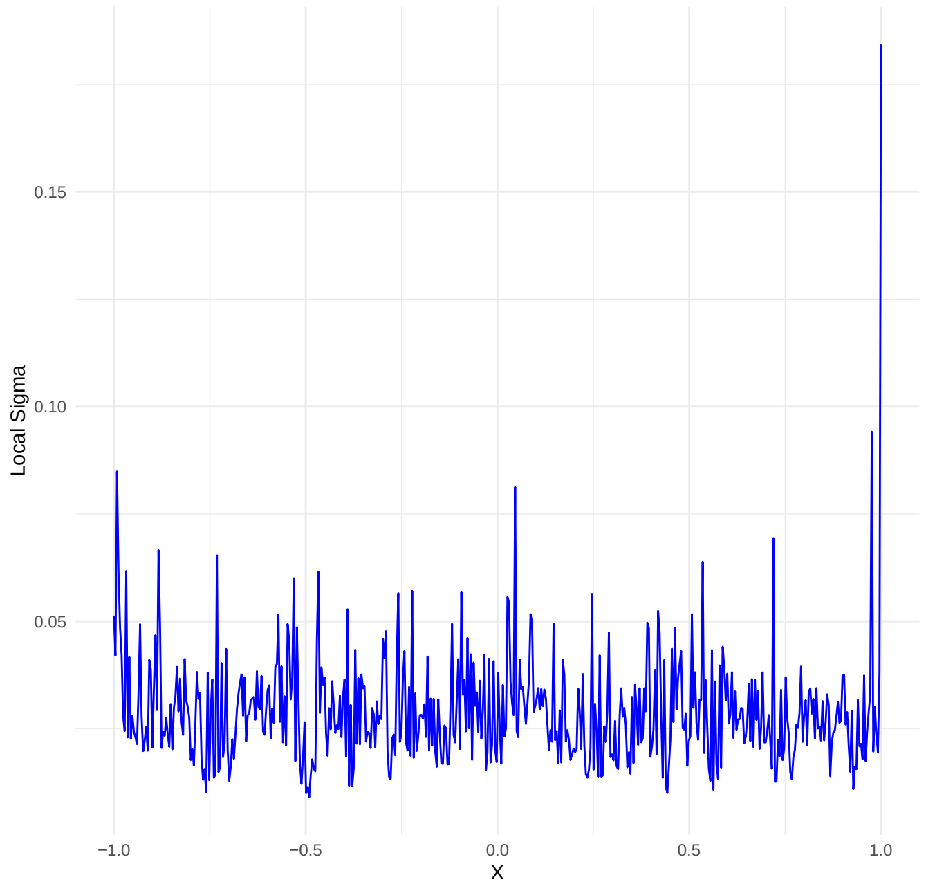
Dataset: s_curve_noise_medium | k= 5 , iter= 21
