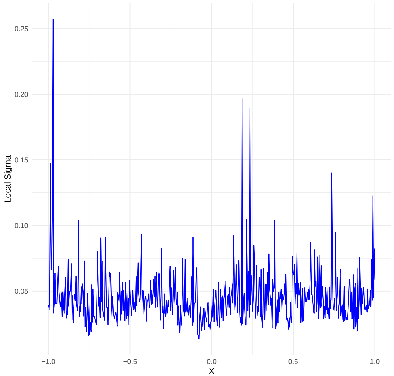
Dataset: s_curve_noise_high | k= 5 , iter= 21
