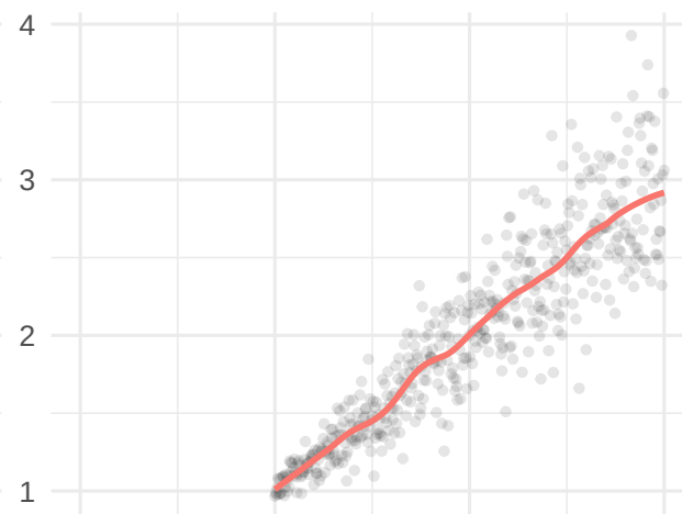
LOESS
