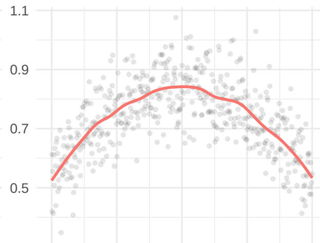
LOESS
