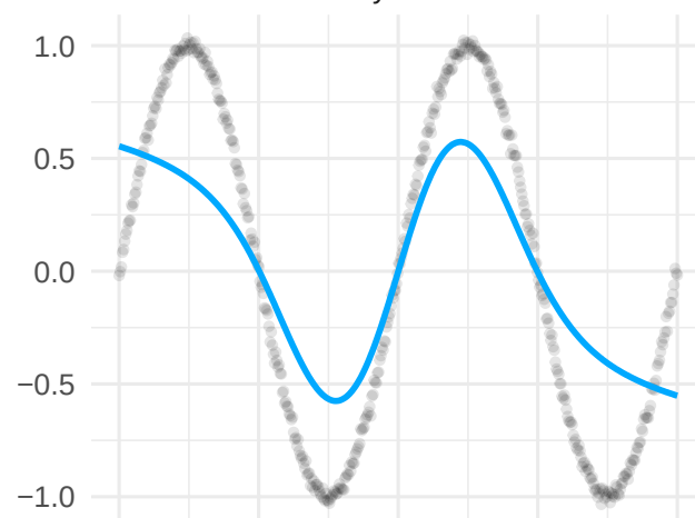
Nadaraya-Watson
