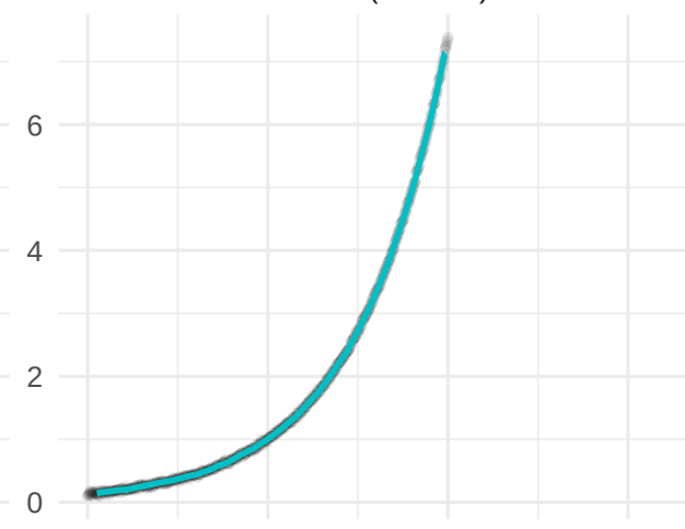
LOESS
