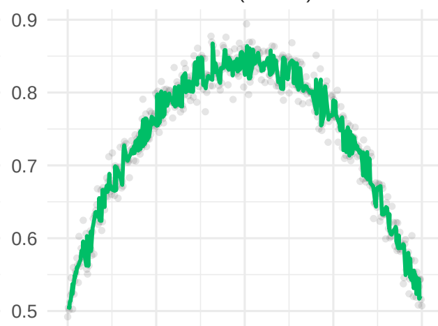
Nadaraya-Watson
