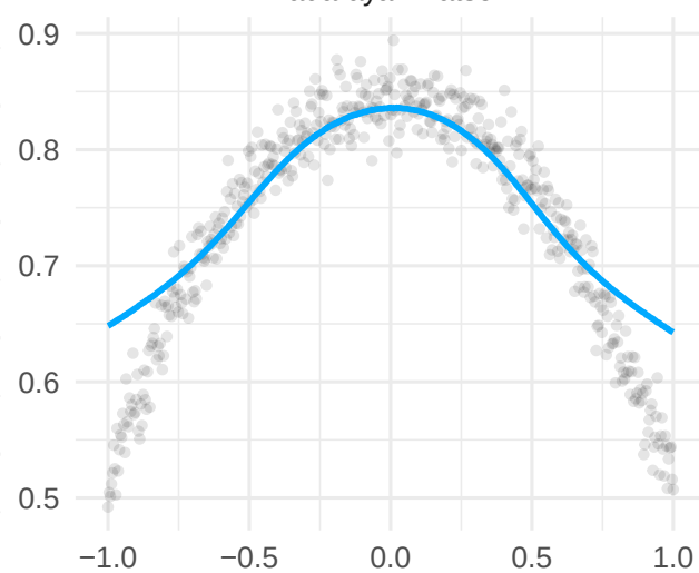
Nadaraya-Watson
