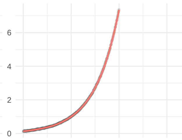
LOESS
