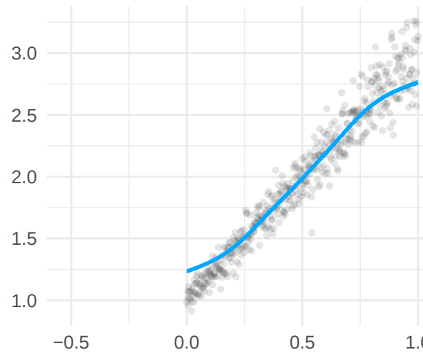
Nadaraya-Watson
