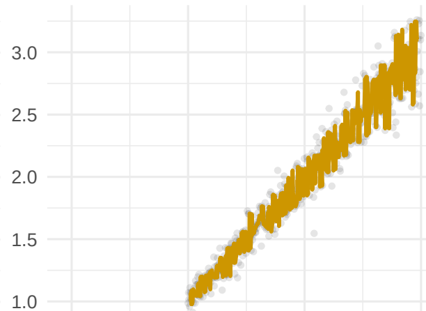
ANWIL
