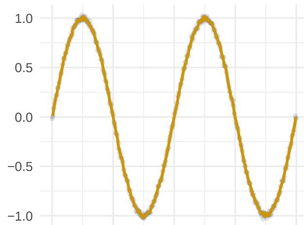
ANWIL
