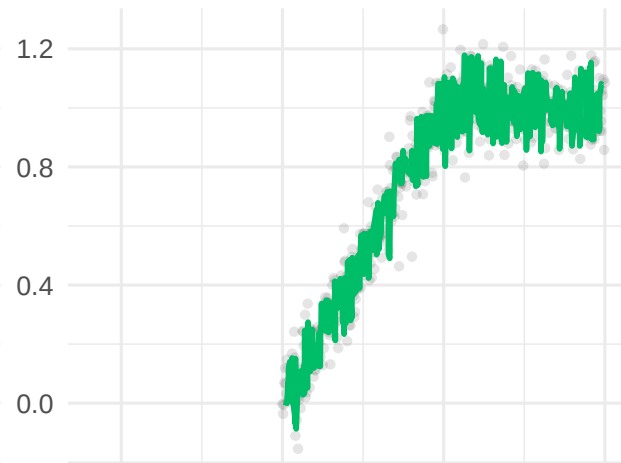
Nadaraya-Watson
