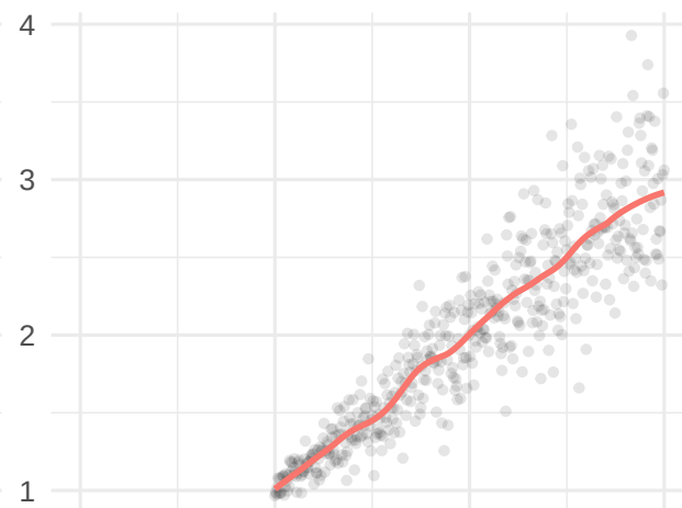
LOESS
