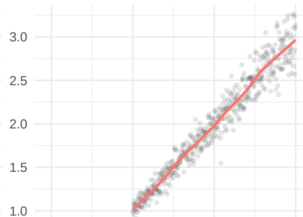
LOESS
