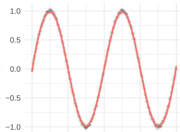
LOESS
