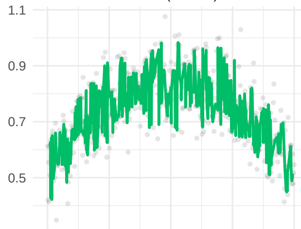
Nadaraya-Watson
