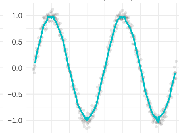
LOESS
