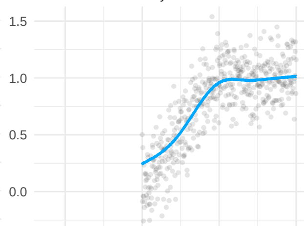
Nadaraya-Watson
