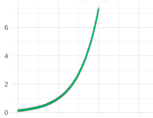
Nadaraya-Watson
