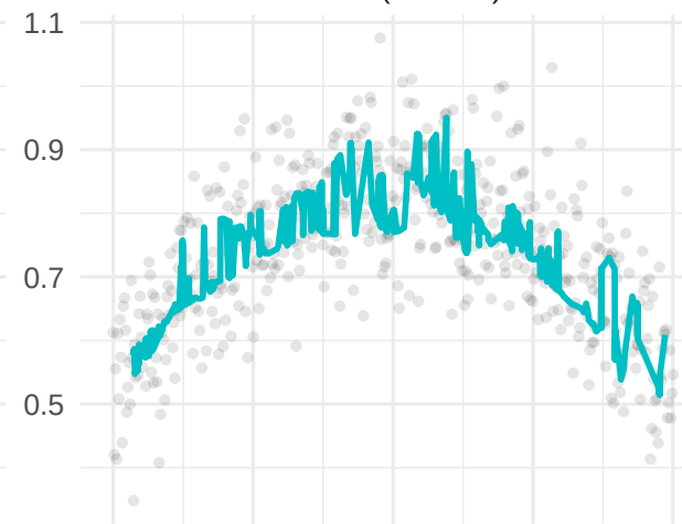
LOESS
