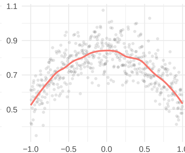
LOESS
