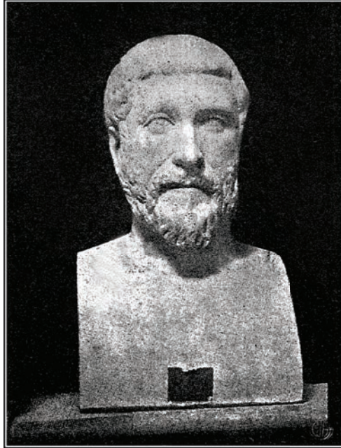
فيثاغورس.
