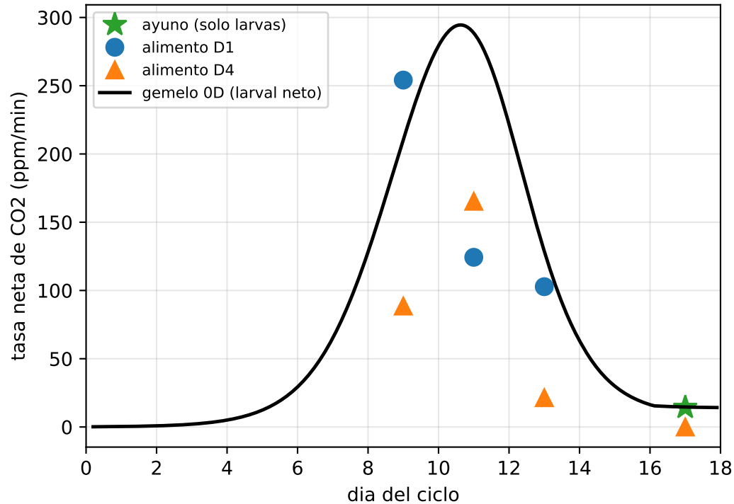
(a) Validación: modelo vs experimento (panera 12.1 L)
