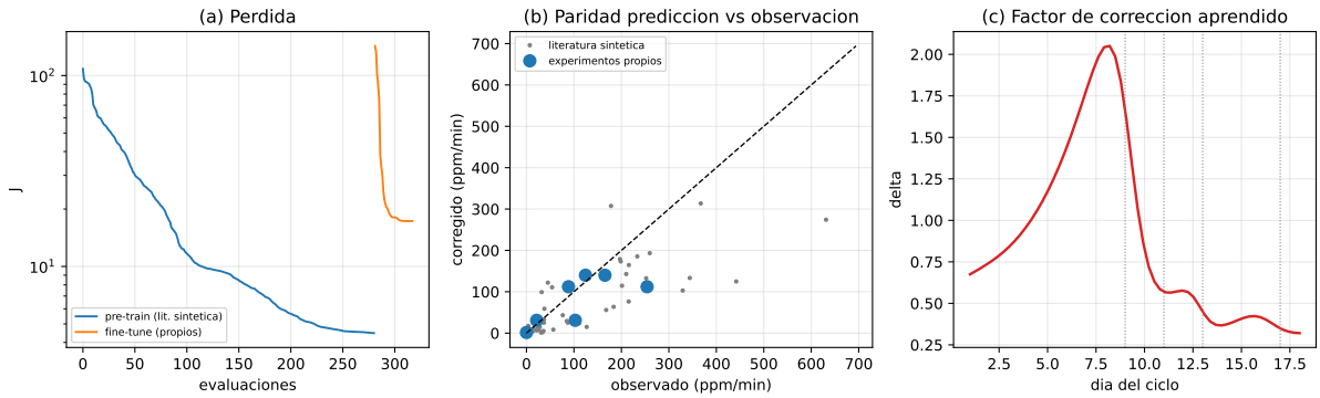
Figura 6: Entrenamiento piloto de la capa PINN. (a) Perdida en el pre-entrenamiento (datos sinteticos tipo literatura) y el ajuste fino (tasas propias). (b) Paridad prediccion corregida vs observacion. (c) Factor de correccion \delta aprendido; las lineas punteadas marcan los dias de medicion.
