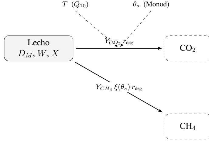
Figura 2: Módulo microbiano del lecho (extensión respecto al modelo de referencia). La constante efectiva k (ec. 6) integra la corrección térmica Q_{10} y la respuesta de humedad tipo Monod; la degradación r_{deg} (ec. 7) crece con la biomasa microbiana X y se apaga al agotarse el sustrato; el CH_4 se activa con la fracción saturada \theta_s via \xi , como indicador cualitativo.
