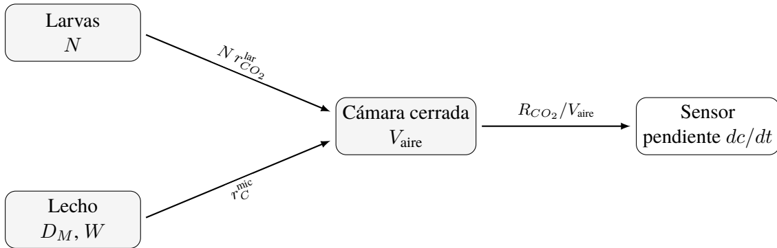
Figura 3: Balance de gas en la cámara estática, sobre el método estándar (Hutchinson y Mosier 1981). Las fuentes larvaria y microbiana acumulan gas en el volumen de aire durante un cierre (ec. 10); el sensor registra la pendiente, llevada a ppm/min con la ley de gas ideal (ec. 11).
