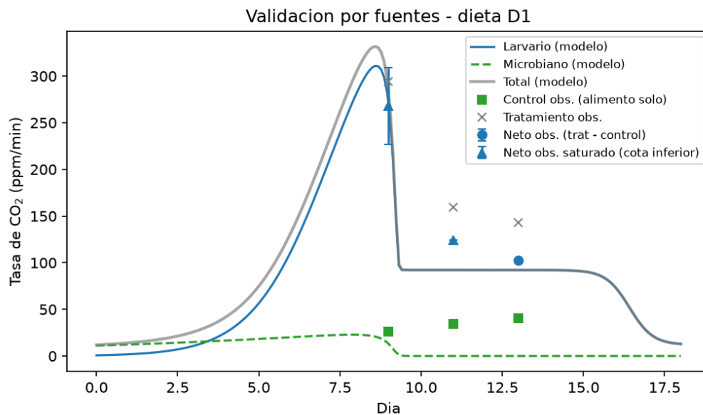
Figura 4: Validación por descomposición de fuentes, dieta D1 (alimento estándar). Curvas: componentes larvaria y microbiana y total del modelo para el régimen de carga única. Puntos: controles de alimento solo (cuadrados), tratamiento (x) y tasa neta tratamiento menos control (círculos; triángulos: cierres saturados, es decir cotas inferiores, con el rango entre cierres).
