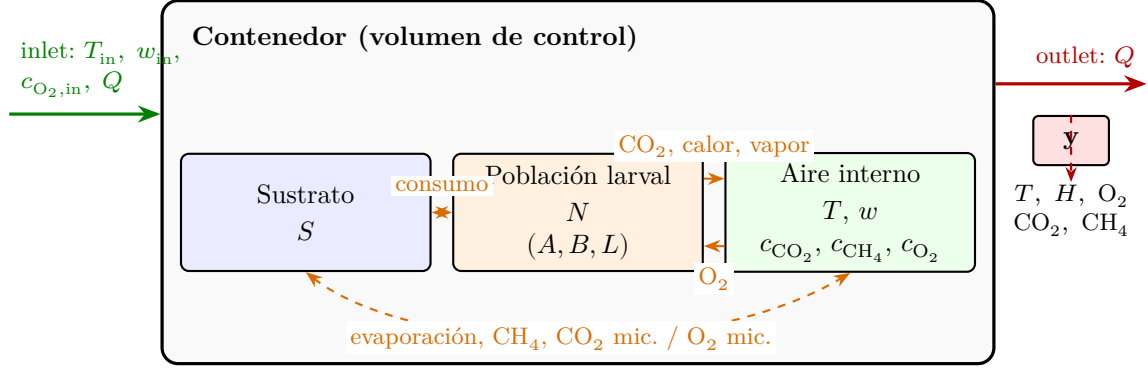
Figura 4: El sistema completo de bioconversión instrumentado (Definición 3.2). Dentro del volumen de control interactúan tres grupos de compartimentos: sustrato, población larval y aire interno; las flechas indican el sentido de cada intercambio (el O_2 fluye del aire hacia larvas y microbiota; el CO_2 , el calor, el vapor y el CH_4 , hacia el aire). La frontera es atravesada únicamente por los flujos de ventilación ( inlet/outlet , caudal Q ); las mediciones y se toman en la corriente de salida y una celda de carga registra la masa total del lote.
