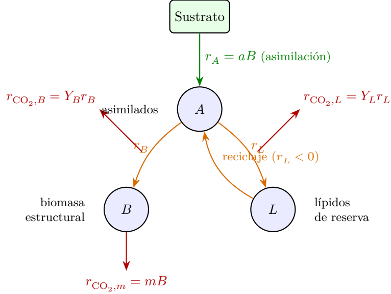
Figura 3: El modelo de Eriksen [2022] como red de compartimentos (Definición 1.3). El sustrato es un forzamiento externo que alimenta el compartimento de asimilados A a tasa r_A = aB ; las flechas internas representan síntesis de biomasa estructural ( r_B ), acumulación de lípidos ( r_L ) y reciclaje de reservas hacia el pool de asimilados cuando r_L < 0 . Las tres flechas rojas son las fuentes de producción de \text{CO}_2 : mantenimiento (proporcional a B ), costo de síntesis estructural y costo de síntesis de lípidos, cuya suma es la producción total (Ec. (7)).
