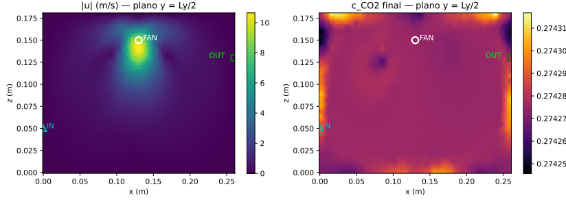
Figura 5: Campo de concentracion (interpolacion IDW sobre cortes) de la camara sellada con ventilador: el trazador inicialmente concentrado en el lecho se homogeneiza en decenas de segundos.
