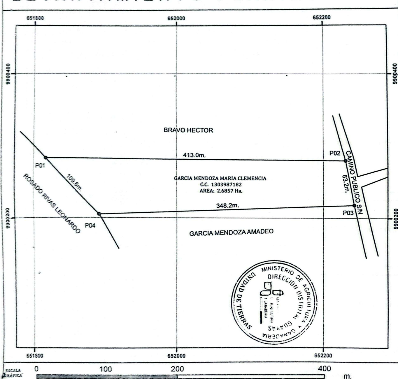
PLANO DE UBICACIÓN GEOGRÁFICA ESCALA 1:50000
